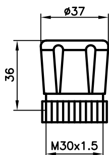
Handregelaufsatz 302H
